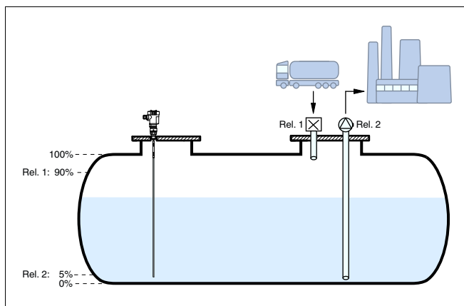
Рис. 11: Пример измерения уровня в горизонтальной цилиндрической емкости
