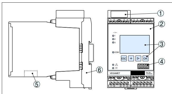
Рис. 1: VEGAMET 624
