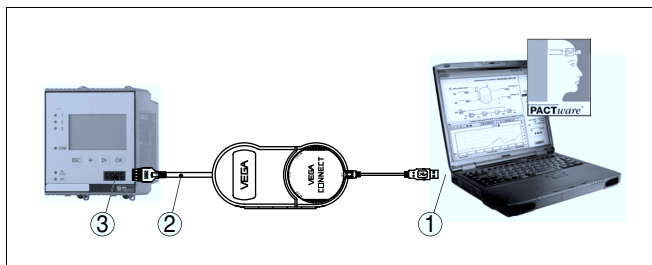
Рис. 6: Подключение через VEGACONNECT
