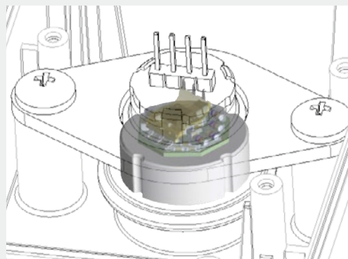
Пример индивидуального решения с керамическим толстопленочным сенсором
