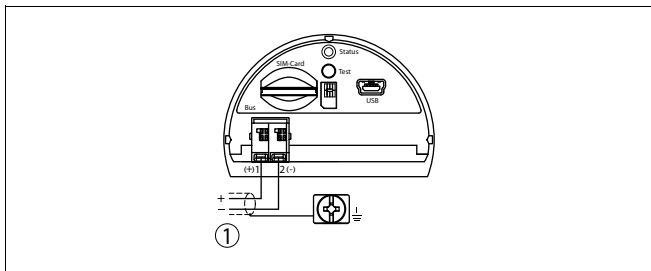
Рис. 28: Подключение модуля мобильной связи к питанию
