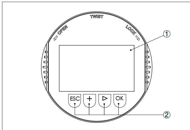
Рис. 35: Элементы индикации и настройки
