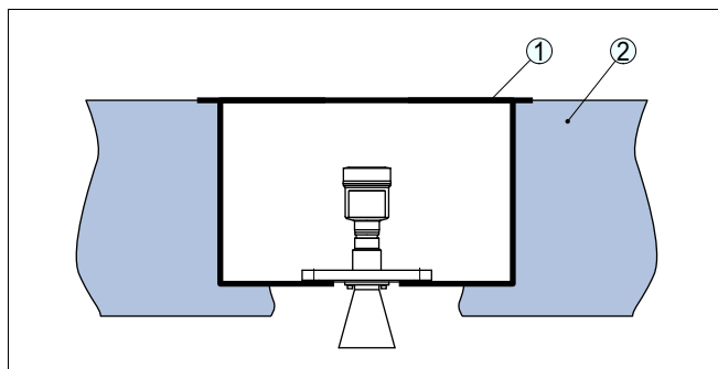
Рис. 19: Монтаж прибора в коробе под полом
