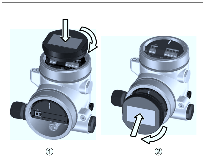
Рис. 34: Установка модуля индикации и настройки в двухкамерном корпусе
