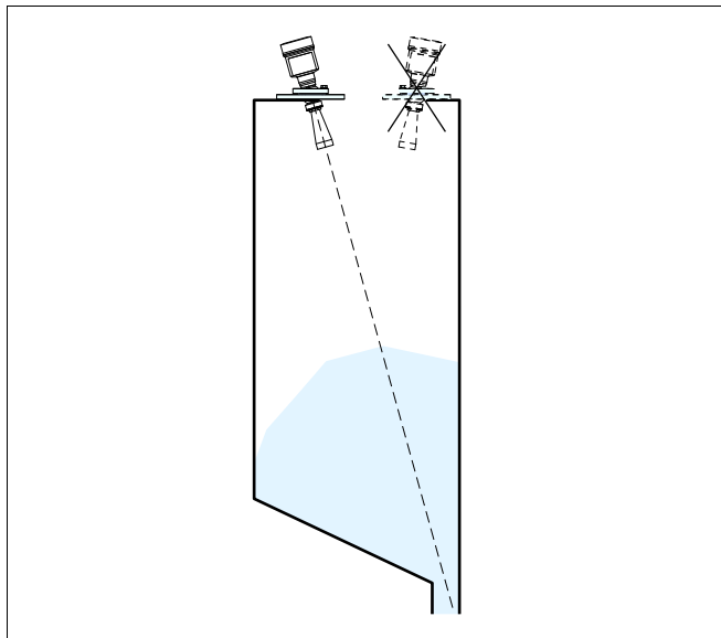
Рис. 21: Ориентация VEGAPULS 68 на выпускное отверстие в центре силоса
