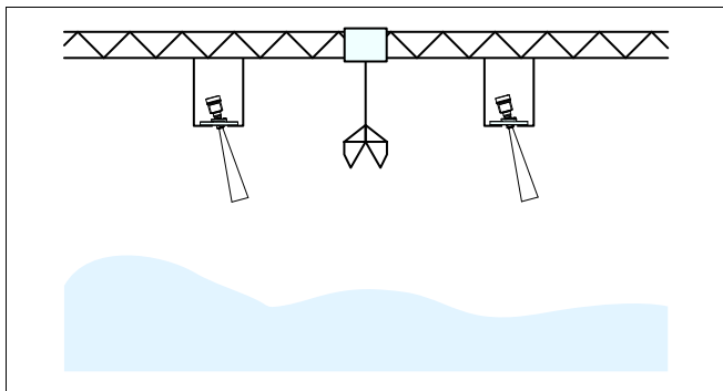
Рис. 17: Радарные датчики на кран-балке
