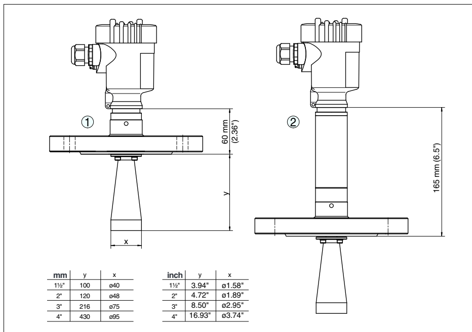
Рис. 58: VEGAPULS 68, с рупорной антенной и фланцевым присоединением
