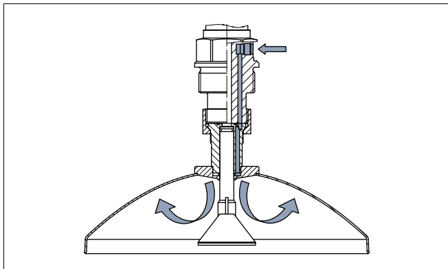
Рис. 23: Вход для подключения продувки параболической антенны
