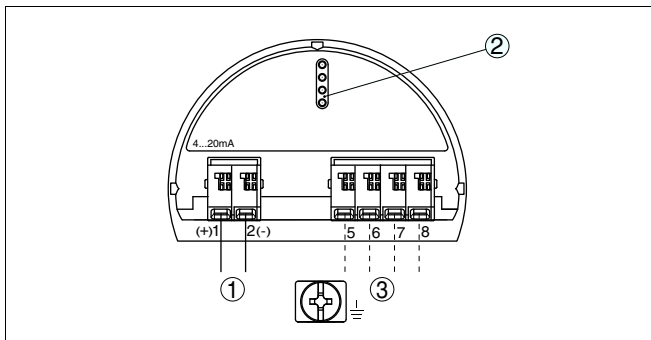
Рис. 29: Отсек электроники (двухкамерный корпус)
