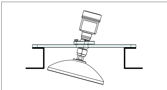
Рис. 11: Расстояние между антенной и патрубком для параболической антенны
