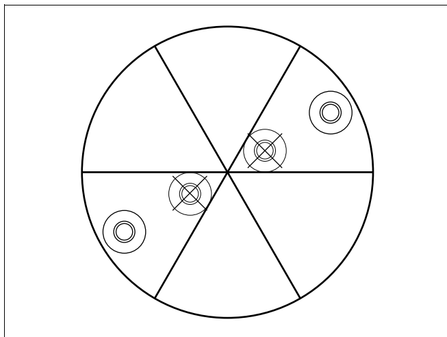
Рис. 20: Монтаж VEGAPULS 68 в многокамерном силосе
