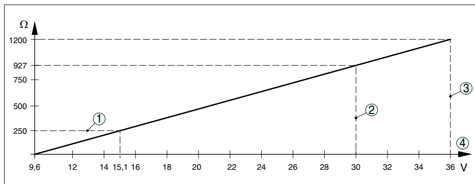
Рис. 51: Диаграмма напряжения
