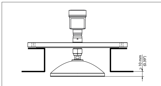
Рис. 9: Рекомендуемые размеры монтажного патрубка для прибора с параболической антенной
