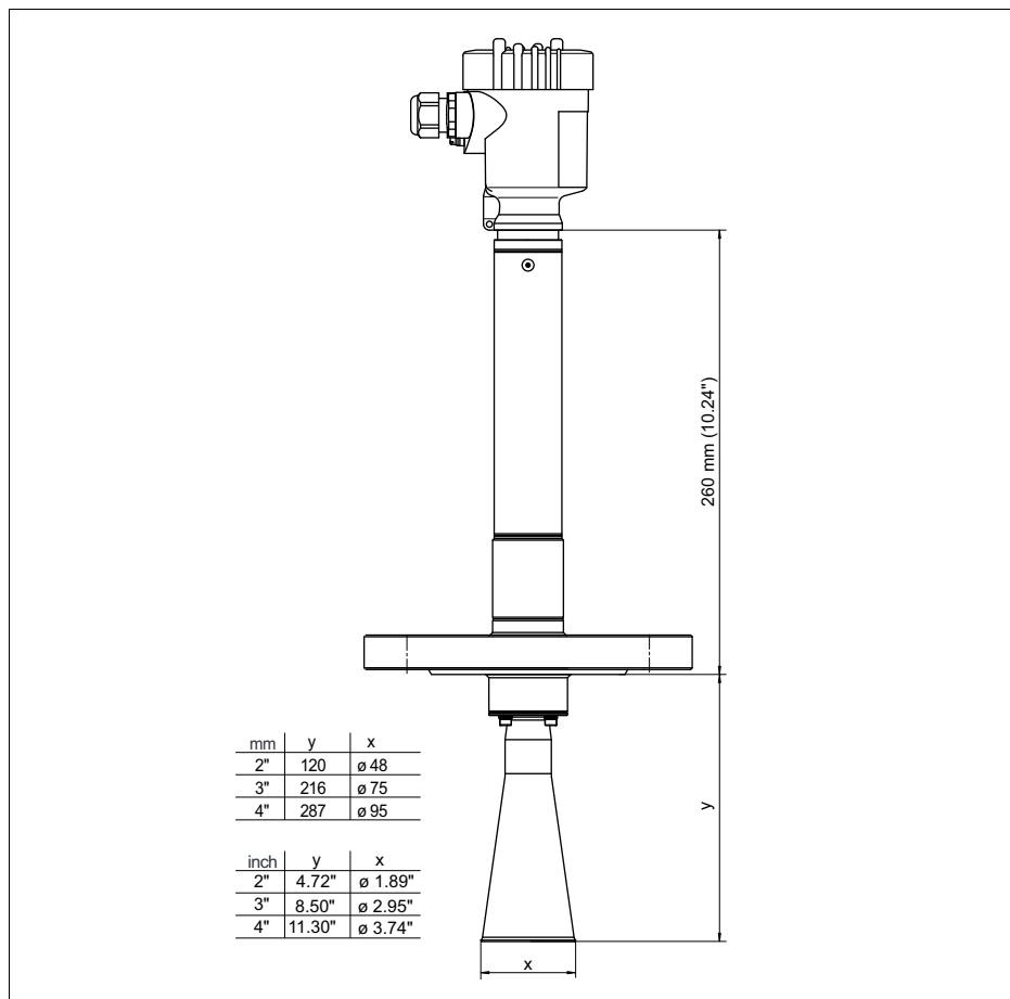
Рис. 59: VEGAPULS 68, с рупорной антенной и фланцевым присоединением, с температурной вставкой до 450 °С
