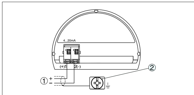
Рис. 30: Отсек подключения (двухкамерный корпус Ex d)
