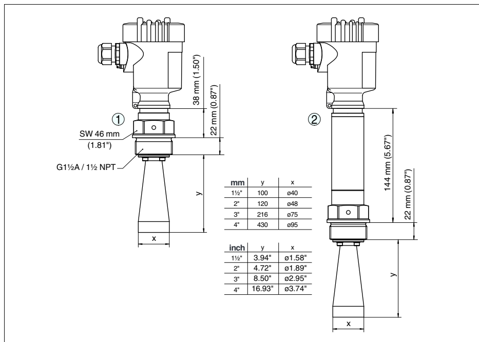
Рис. 57: VEGAPULS 68 с рупорной антенной и резьбовым присоединением
