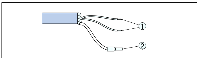
Рис. 32: Назначение проводов постоянно подключенного соединительного кабеля
