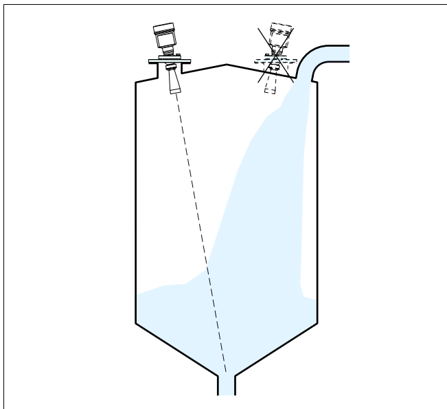
Рис. 7: Монтаж радарного датчика при втекающем продукте
