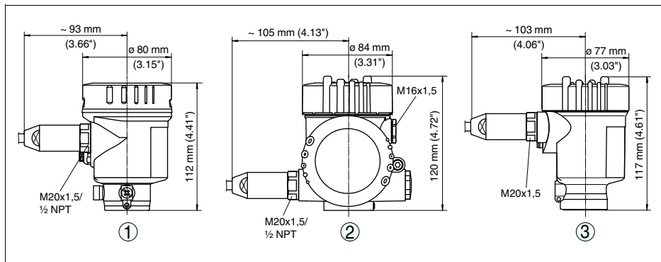
Рис. 56: Корпуса в исполнении IP 66/IP 68 (1 bar) - с установленным модулем индикации и настройки корпус выше на 9 мм/0.35 in
