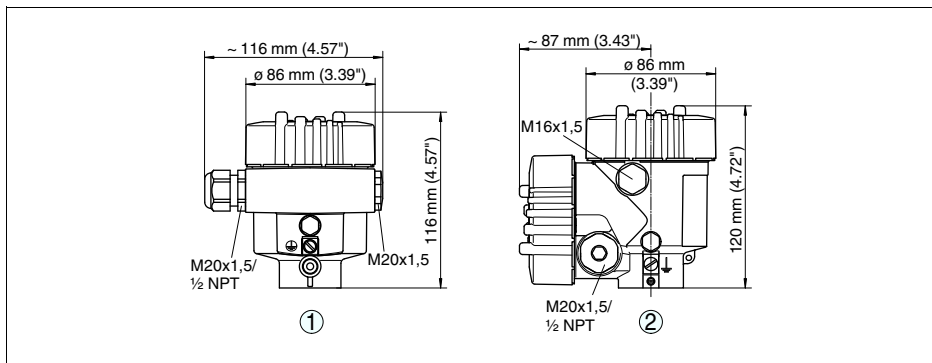
Рис. 53: Корпуса в исполнении IP 66/IP 68 (0,2 bar) - с установленным модулем индикации и настройки корпус выше на 9 мм/0.35 in
