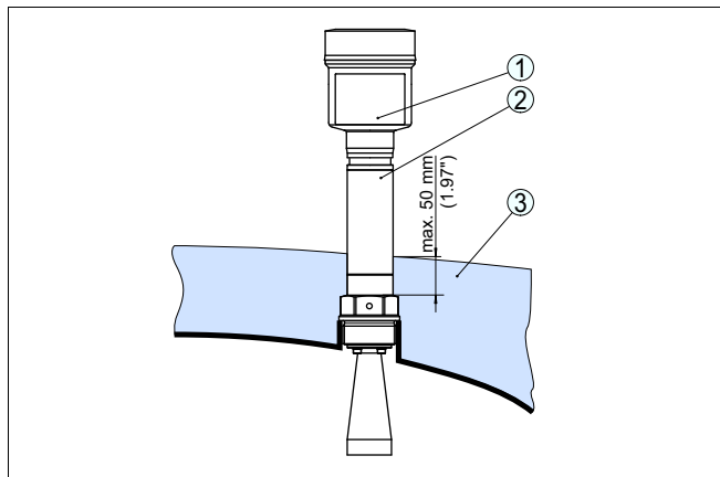
Рис. 18: Монтаж устройства на емкости с термоизоляцией
