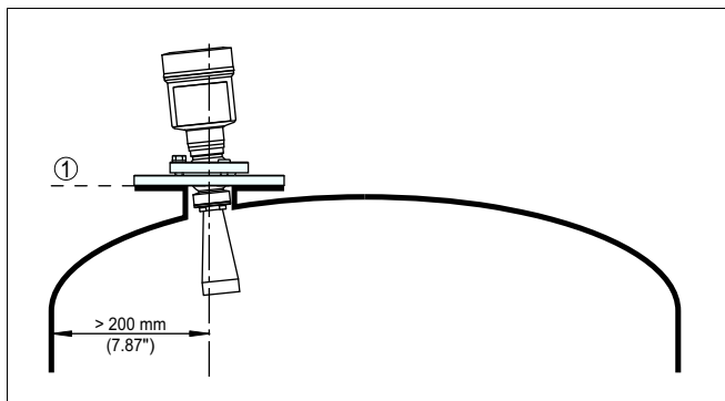
Рис. 6: Монтаж радарного датчика на округлой крыше емкости
