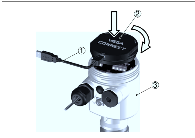
Рис. 36: Подключение ПК через интерфейсный адаптер прямо к датчику
