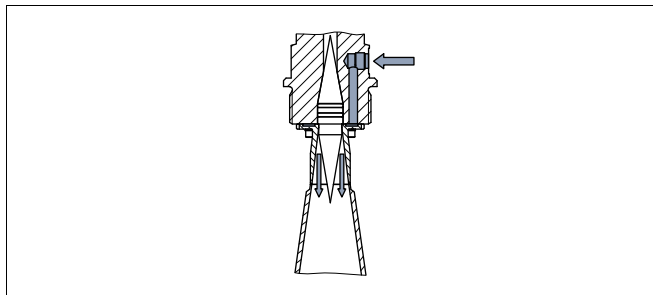
Рис. 22: Вход для подключения продувки рупорной антенны
