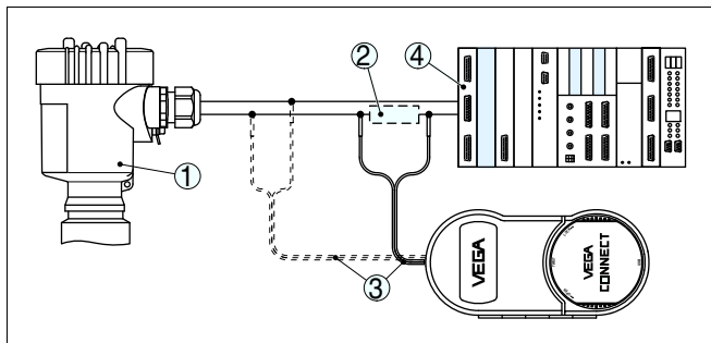
Рис. 37: Подключение ПК к сигнальному кабелю через HART
