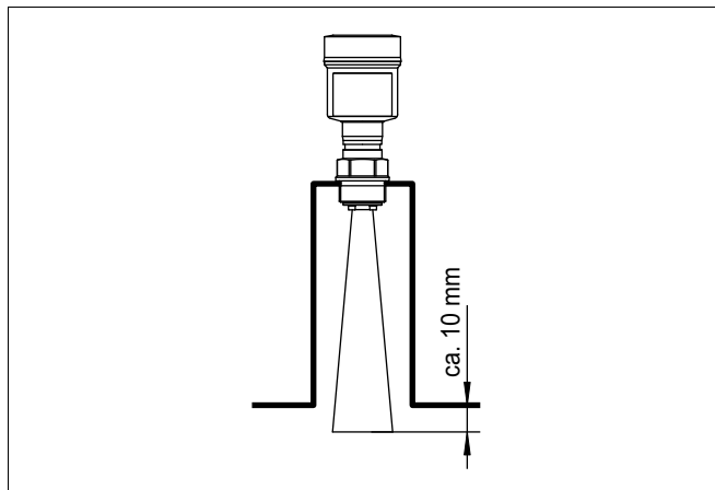
Рис. 8: Рекомендуемые размеры монтажного патрубка для прибора с рупорной антенной
