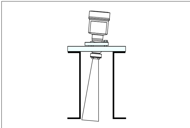
Рис. 10: Расстояние между антенной и патрубком для рупорной антенны
