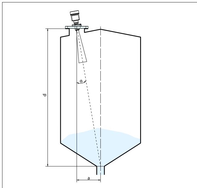
Рис. 14: Рекомендация по монтажу VEGAPULS 68 с наклоном
