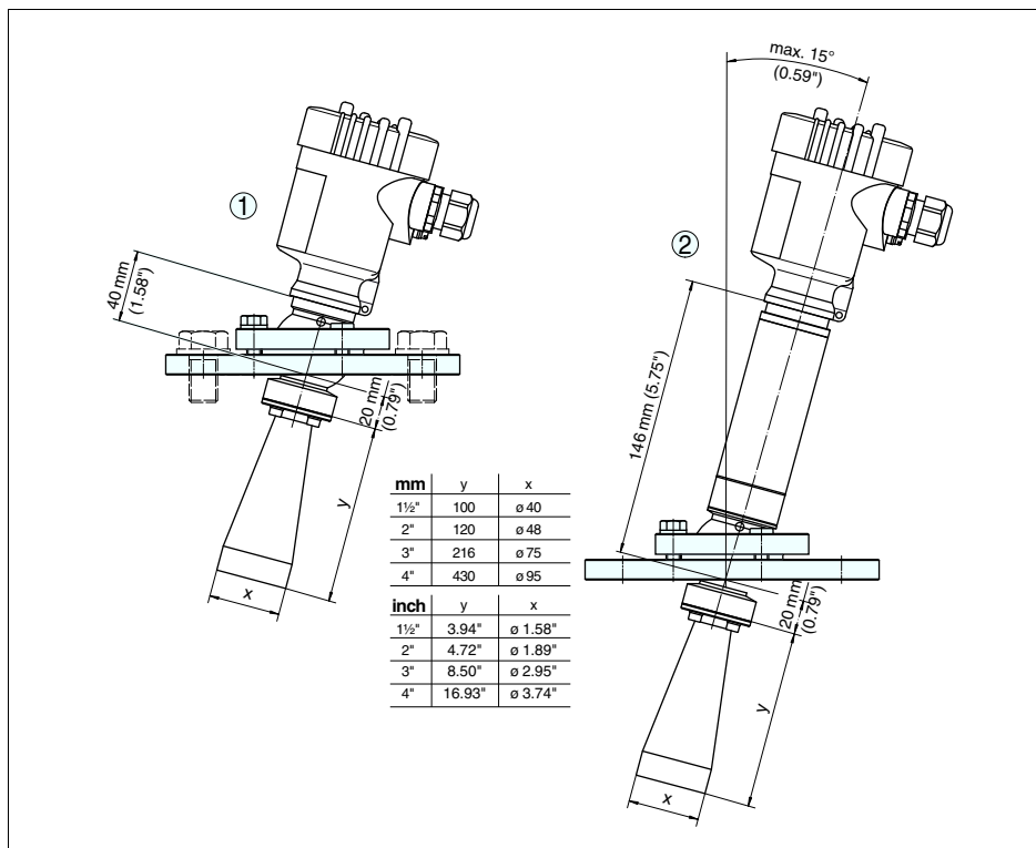
Рис. 60: VEGAPULS 68, с рупорной антенной и поворотным креплением
