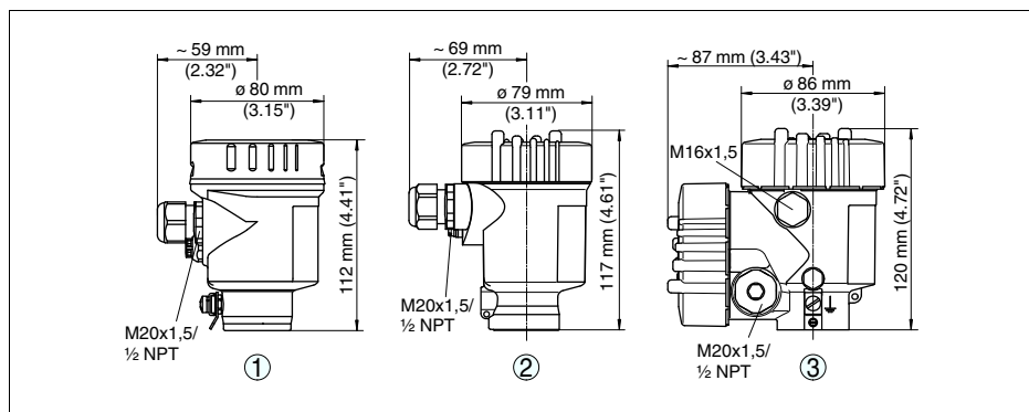
Рис. 55: Корпуса в исполнении IP 66/IP 68 (0,2 bar) - с установленным модулем индикации и настройки корпус выше на 9 мм/0.35 in
