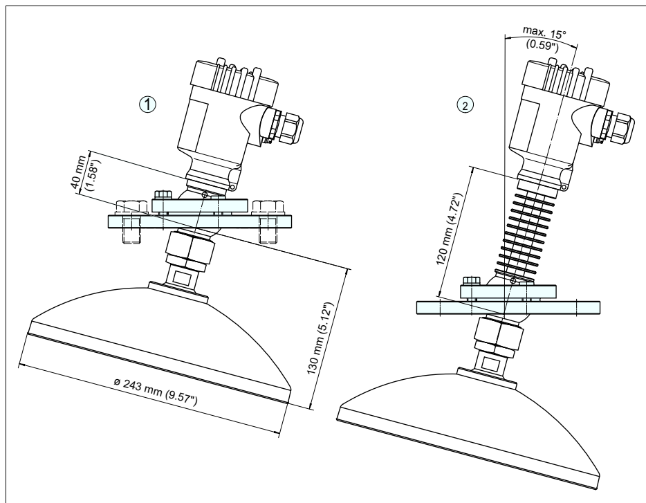
Рис. 61: VEGAPULS 68, с параболической антенной и поворотным креплением
