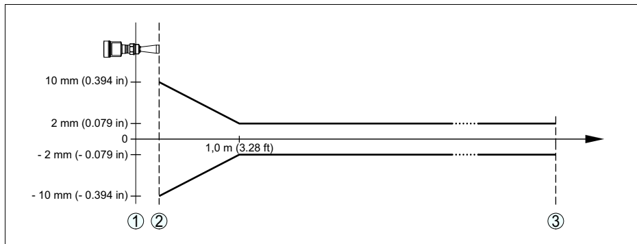
Рис. 50: Погрешность измерения при эталонных условиях
