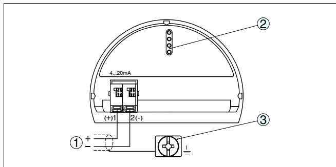
Рис. 27: Отсек подключения (двухкамерный корпус)
