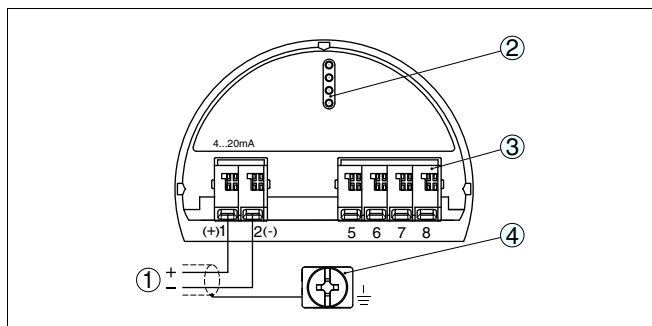
Рис. 25: Отсек электроники и подключения - однокамерный корпус
