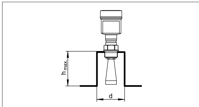
Рис. 12: Ориентировочные размеры патрубков
