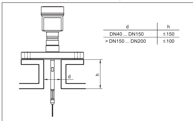
Рис. 9: Монтажный патрубок
