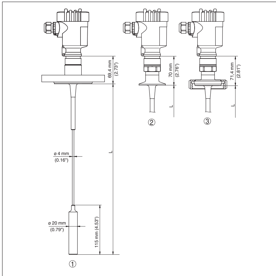
Рис. 54: VEGAFLEX 83, тросовое исполнение с натяжным грузом
