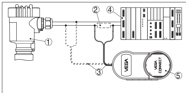
Рис. 30: Подключение ПК к сигнальному кабелю через HART
