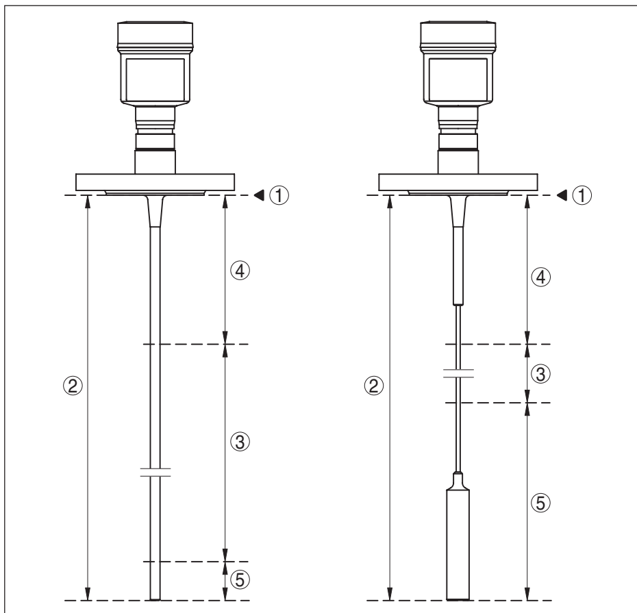
Рис. 43: Диапазоны измерения - VEGAFLEX 83
