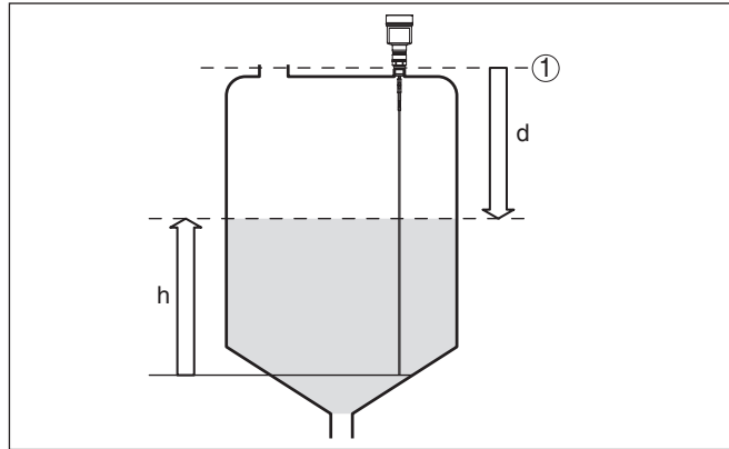
Рис. 5: Измерение уровня
