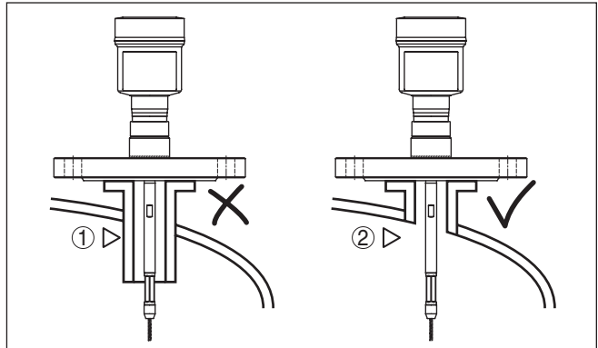
Рис. 10: Патрубок монтируется заподлицо
