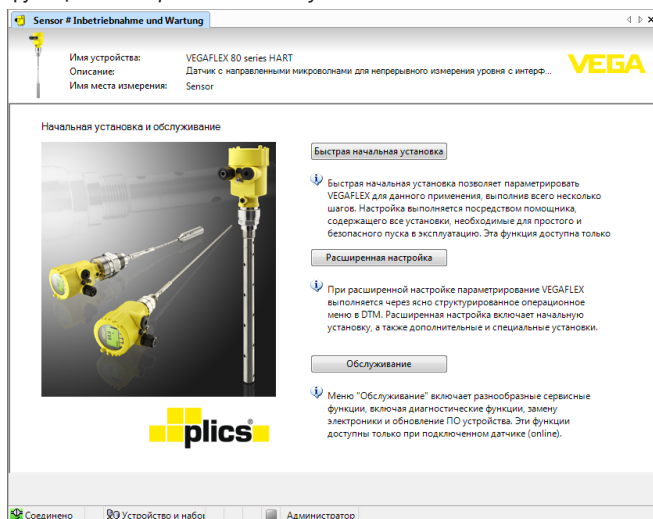
Рис. 32: Выбор Быстрой начальной установки
