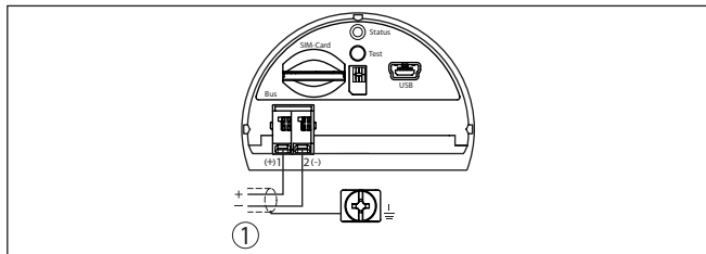
Рис. 17: Отсек подключения (модуль PLICSMOBILE)
