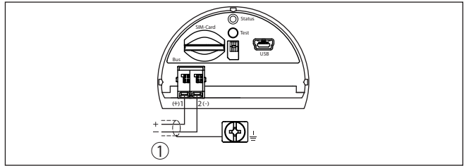
Рис. 24: Отсек подключения встроенного модуля мобильной связи PLICSMOBILE
