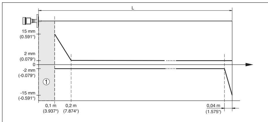
Рис. 44: Погрешность измерения VEGAFLEX 83 в стержневом исполнении с покрытием (продукт - вода)
