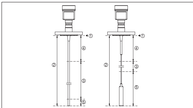
Рис. 3: Диапазоны измерения - VEGAFLEX 83
