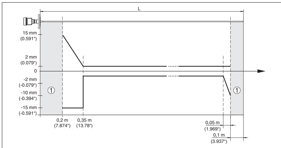
Рис. 45: Погрешность измерения VEGAFLEX 83 в стержневом исполнении с покрытием (продукт - масло)
