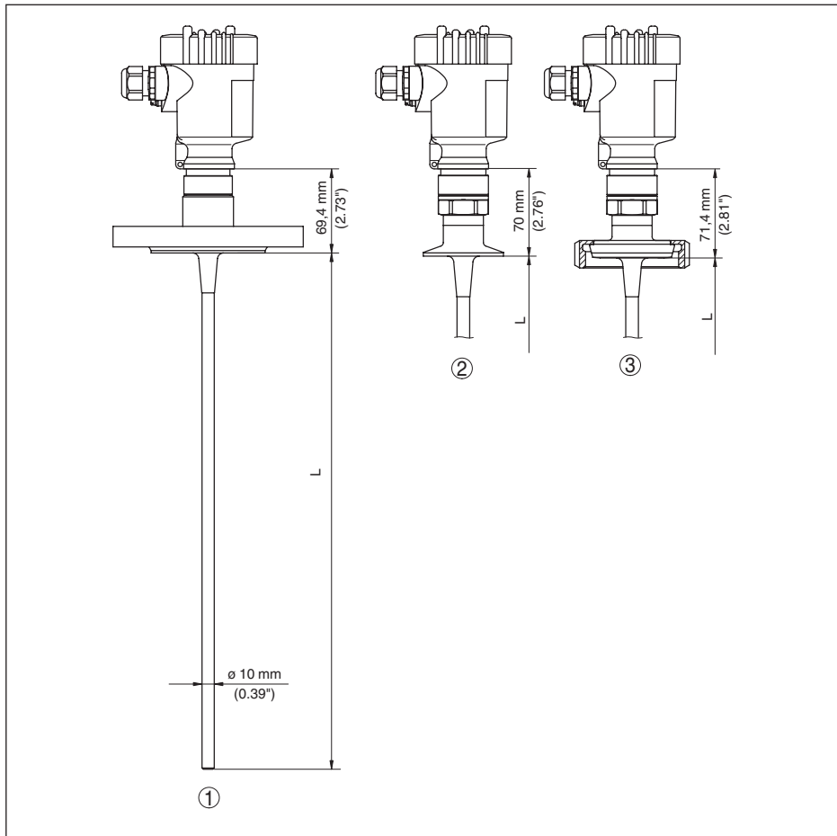
Рис. 55: VEGAFLEX 83, стержневое исполнение
