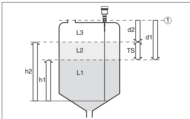
Рис. 6: Измерение межфазного уровня
