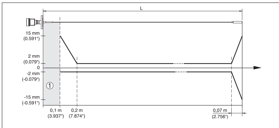
Рис. 46: Погрешность измерения VEGAFLEX 83 в тросовом исполнении с покрытием (продукт - вода)
