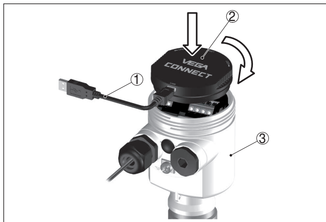
Рис. 29: Подключение ПК через интерфейсный адаптер прямо к датчику
