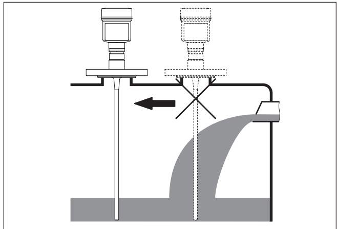
Рис. 11: Монтаж датчика при втекающем продукте
